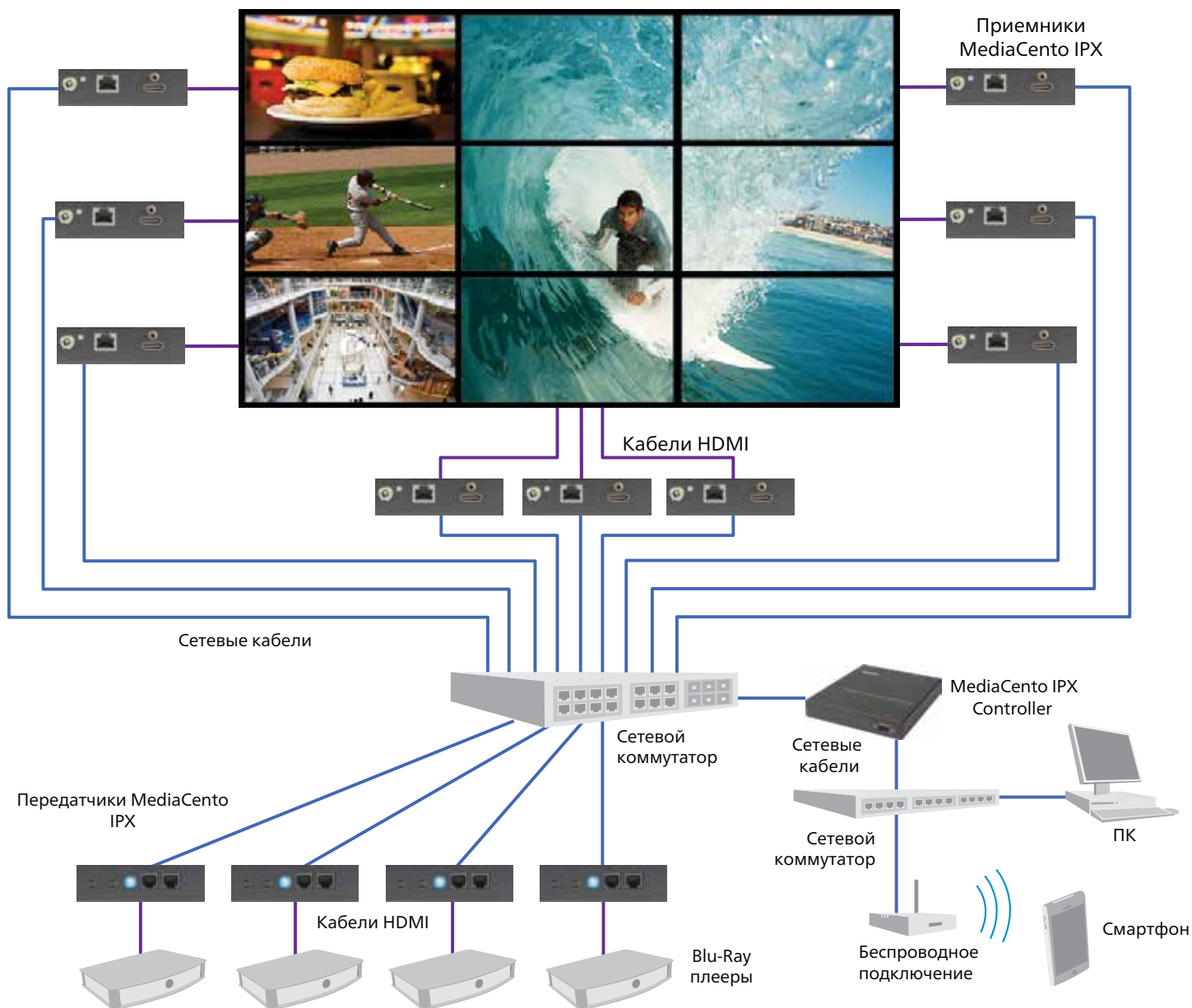
Видеостена 3x3
